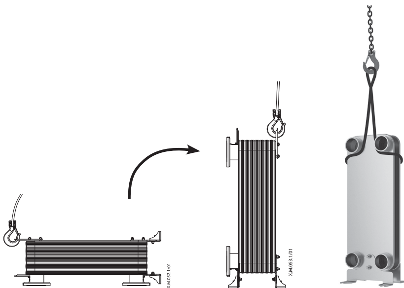
Fig. 2 Løft / Fig. 2 Lifting / Abb. 2 Heben / Fig. 2 Levage / Fig. 2 Elevación / Fig. 2 Sollevamento / Fig. 2 Lyftning / Fig. 2 Hljsen / Kuva 2 Nostaminen / 2 pav. Kėlimas / 2. att. Pacelšana / Joonis 2 Tõstmine / Obr. 2 Zdvíhanie / Slika 2 Dviganje / SI. 2 Podizanje / 图 2 起吊 / Фуз. 2 Повдигане / Slika 2 Podizanje / Fig. 2 Ridicare / 2. ábra: Emelés / Obr. 2 Zvedáni / Rys. 2 Podnoszenie / Рис. 2 Подъем
