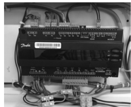
Bild 4: Tillfälliga anslutningar
