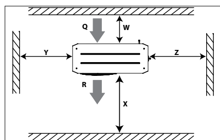
Afbeelding 1: Minimale plaatsingsafstand
