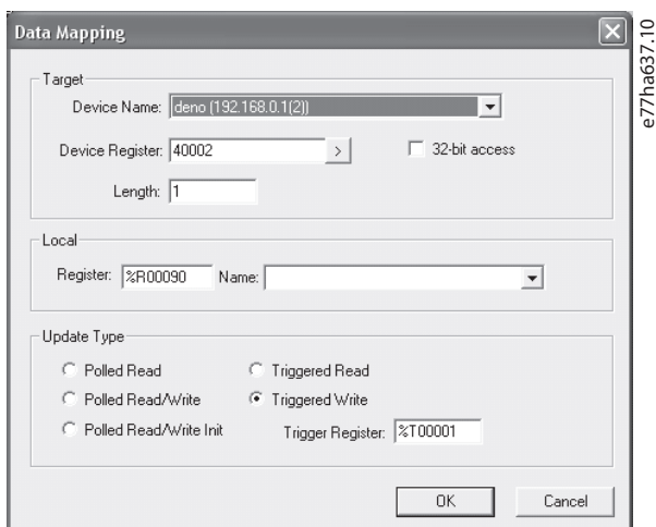
Рисунок 7.6 Отправка команды пуска (регистр 40002)
