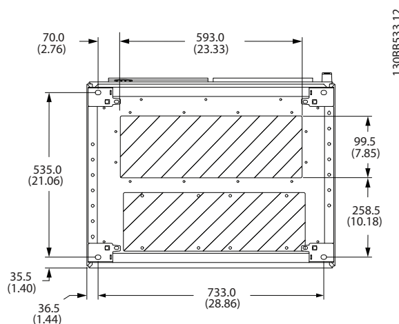
Рисунок 3.24 F8, кабельный ввод преобразователя частоты (вид снизу)
