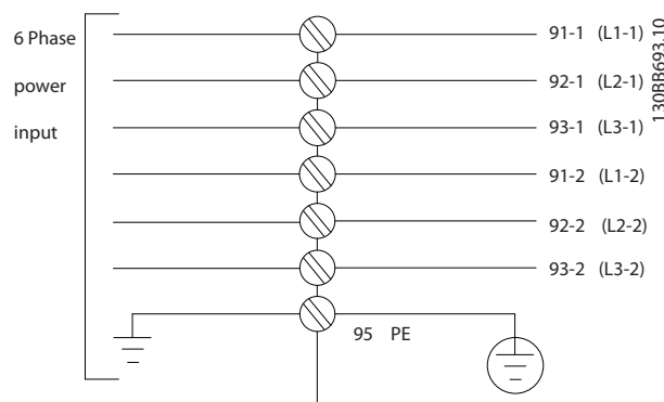
Рисунок 3.32 Подключение кабеля электропитания
