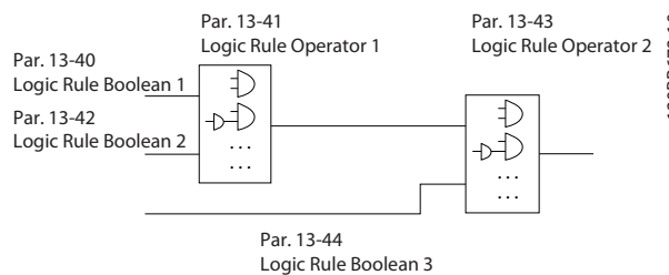
Рисунок 5.6 Логические соотношения
