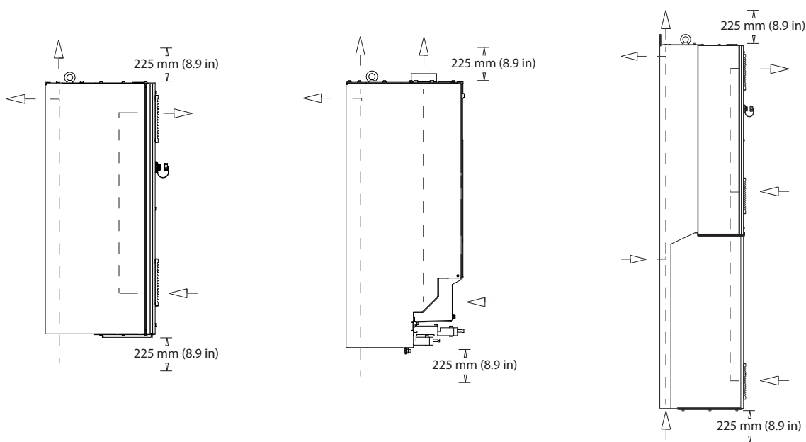
Рисунок 5.10 Стандартная конфигурация воздушной циркуляции для корпусов D1h/D2h (слева), D3h/D4h (посередине) и D5h–D8h (справа).
