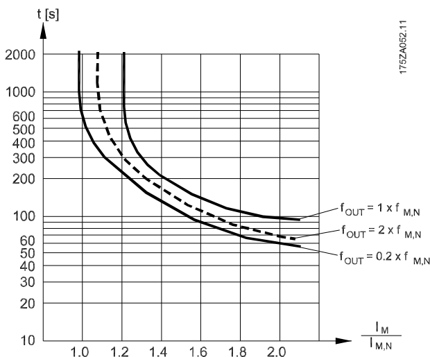
Рисунок 5.1 Характеристики ЭТР
