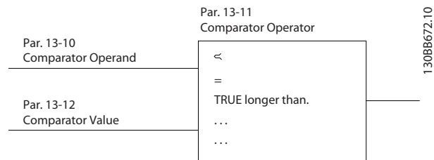
Рисунок 5.5 Компараторы
