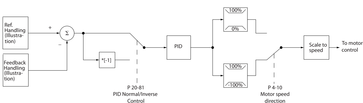
Рисунок 11.7 Блок-схема регулятора с замкнутым контуром
