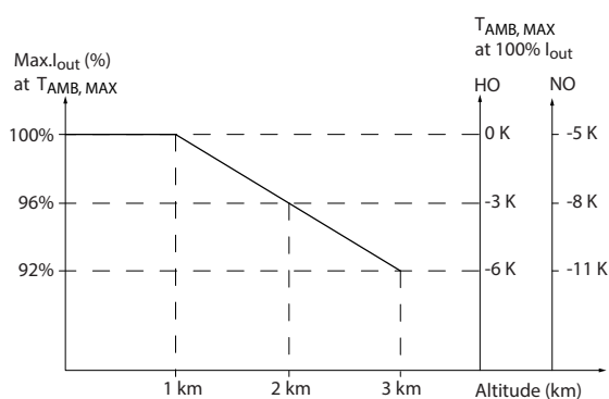
Рисунок 9.2 Снижение выходного тока в зависимости от высоты над уровнем моря при температуре окружающей среды T_{AMB,MAX}
