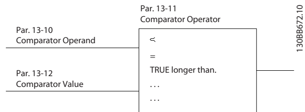
Рисунок 5.5 Компараторы
