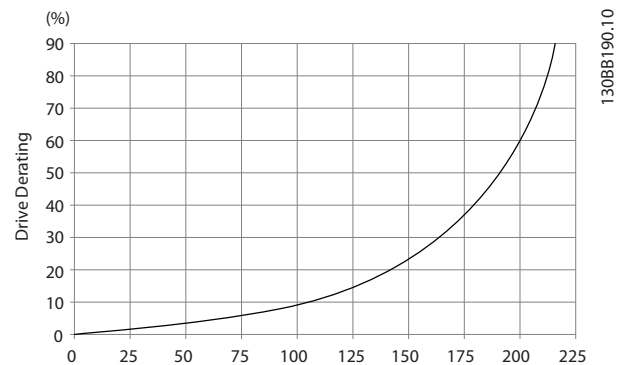
Рисунок 9.7 Снижение номинальных характеристик в зависимости от изменения давления для корпусов F1–F4. Циркуляция воздуха: 580 куб. футов/мин (985 м³/ч)
