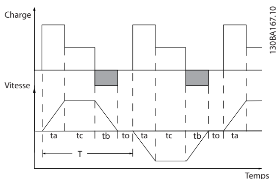
Рисунок 10.21 Типичный цикл торможения
