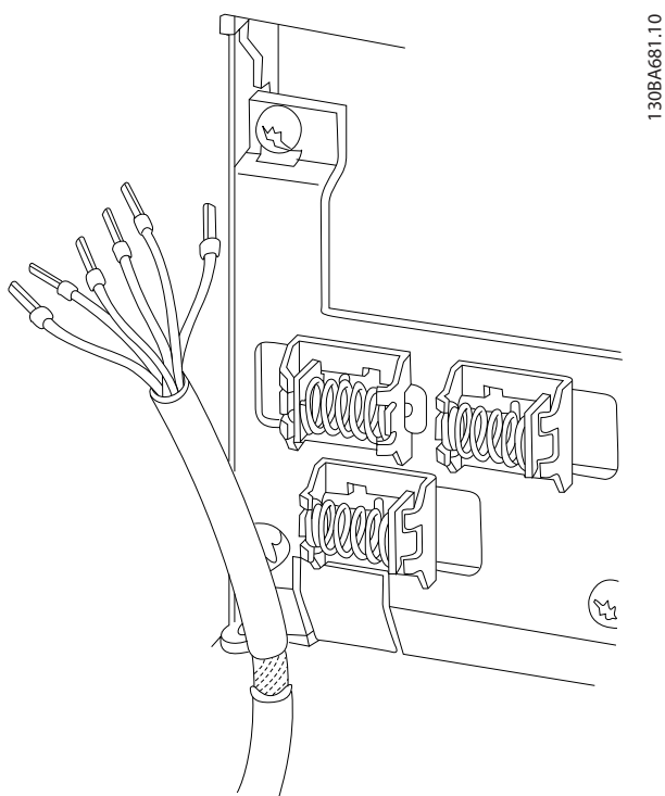
Рисунок 10.16 Заделка экрана и разгрузка натяжения кабеля управления
