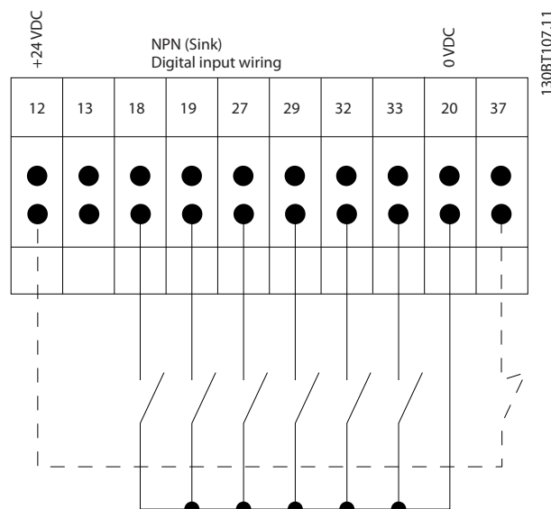
Рисунок 10.15 Входная полярность клемм управления (NPN-сток)
