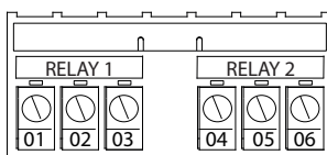
Рисунок 10.13 Клеммы реле 1 и реле 2
