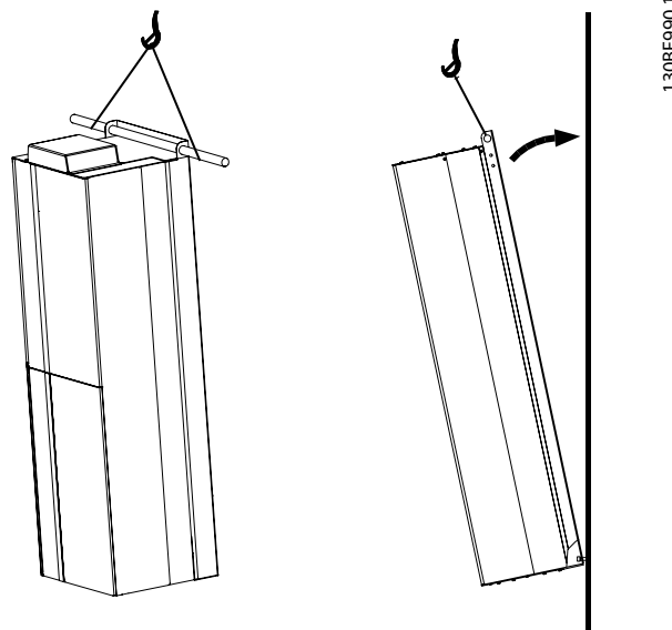
Рисунок 9.1 Рекомендуемый способ подъема для корпусов E1–E2
