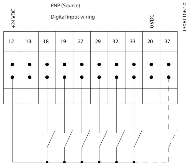
Рисунок 10.14 Входная полярность клемм управления (PNP-источник)
