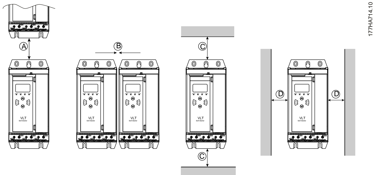
Рисунок 4: Зазоры
