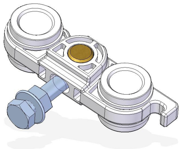
Рис. 16: Роликовый аппарат
