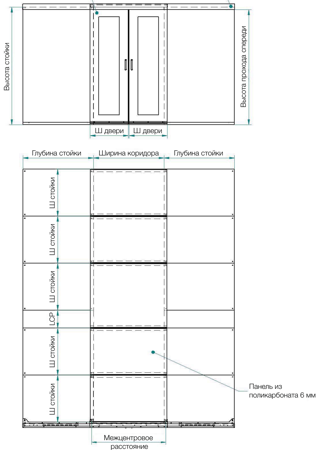
Рис. 7: План установки (пример)
