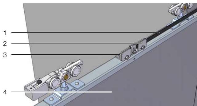
Рис. 34: Крепление зубчатого ремня на правой двери
