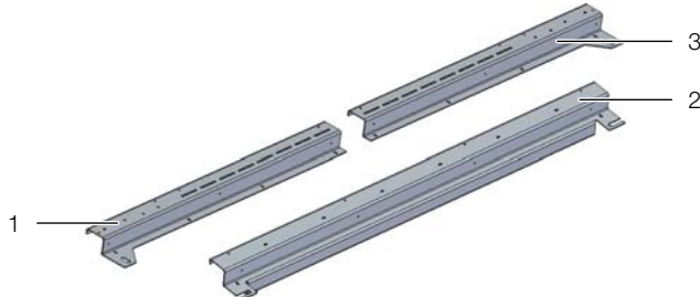
Рис. 11: Крепежные рейки
