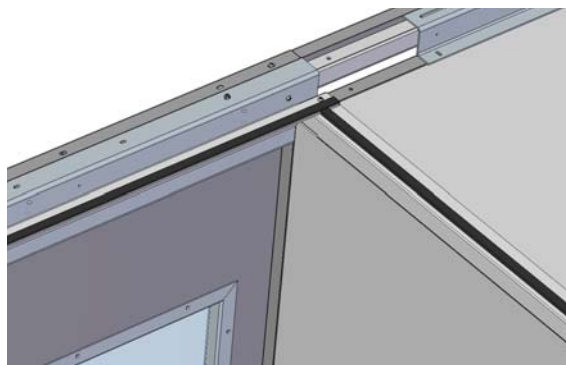
Рис. 50: Нанесение уплотнения
