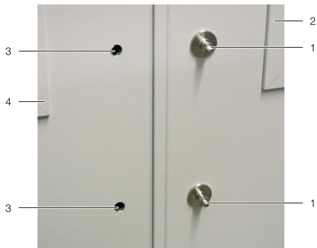
Рис. 31: Закрепление ручки двери
