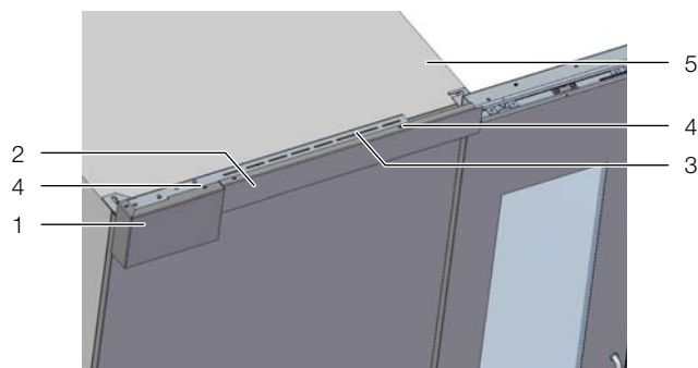
Рис. 44: Монтаж кожуха шкива и панели
