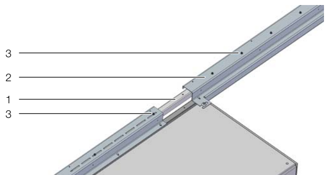
Рис. 14: Крепление направляющей шины на направляющей рейке
