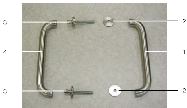
Рис. 30: Отдельные компоненты ручки двери
