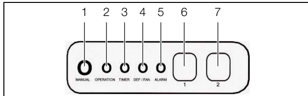
Рис. 16: Элемент управления и индикации 3
