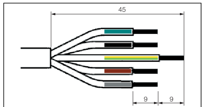
Рис. 9: Размеры снимаемой изоляции кабеля и отдельных проводов
