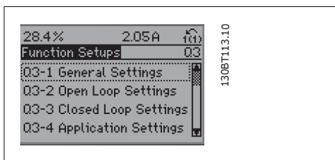
Рисунок 1.10: Операция 4. Появляется меню настройки функций. Выберите Q3-1 Общие настройки. Нажмите [OK].
