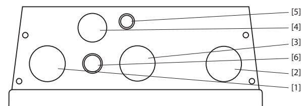
Рисунок 4.5 B1 (IP55)
