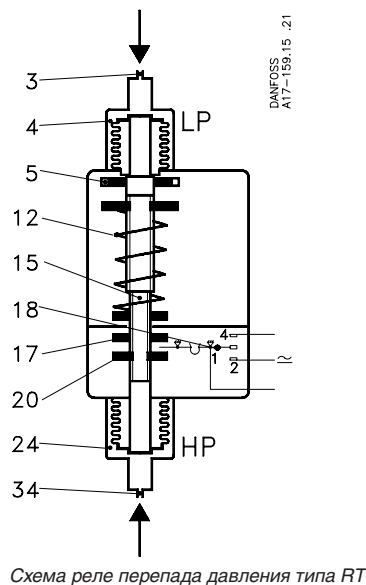
Схема реле перепада давления типа RT
