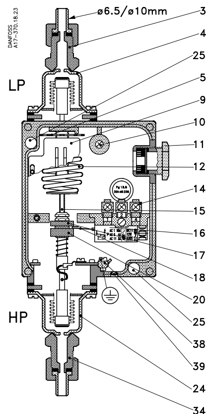
Реле перепада давления типа RT
