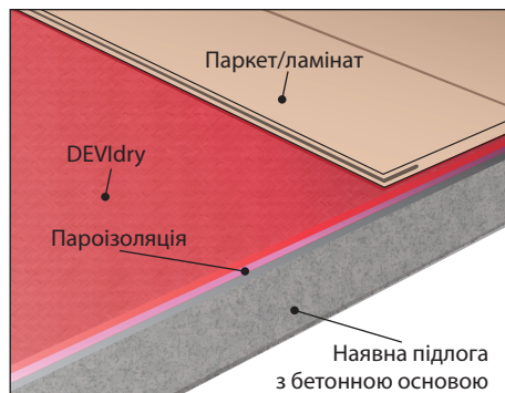
Покриття підлоги DEVIdry™ 55 або 100 Конструкція бетонної підлоги
