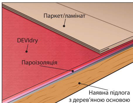
Покриття підлоги DEVIdry™ 55 Конструкція дерев'яної підлоги
