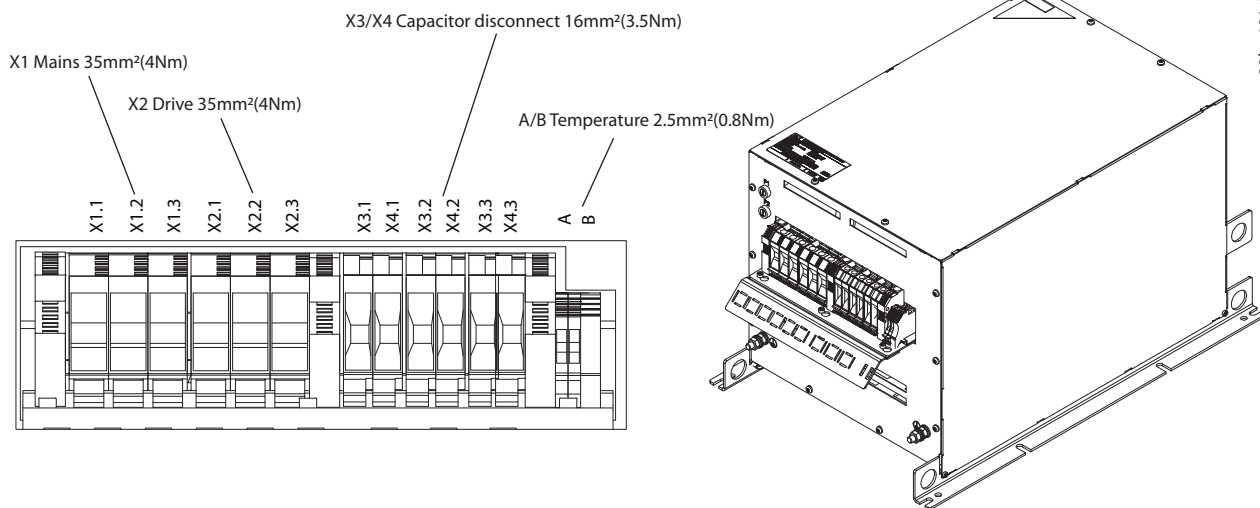
Рисунок 7.15 IP20 X4-V3, внутренний вентилятор, обозначения клемм и 3D-вид
