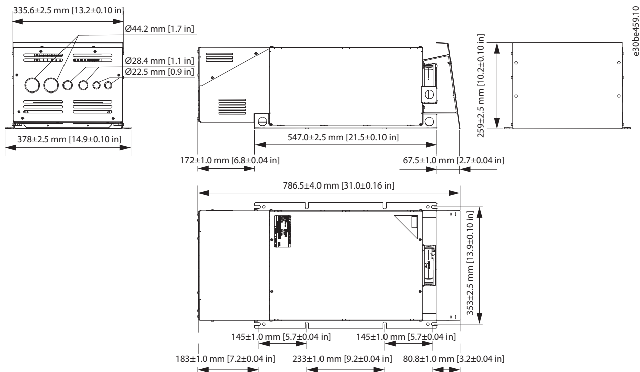
Рисунок 7.38 IP21 X3-V3, внутренний и внешний вентилятор
