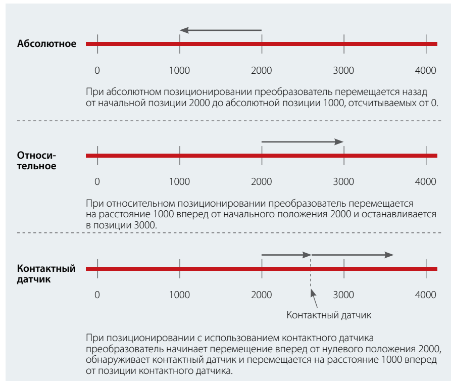
Рис. 3. ИМС поддерживает три режима позиционирования
