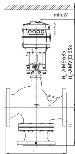
AMV(E) 65x, AMV 685 + VF 2, VF 3 (DN 125, 150)
