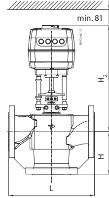
AMV(E) 65x + VL 2, VL 3 (DN 100)
