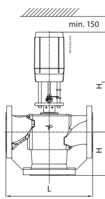
AMV(E) 55, 56 + VL 2, VL 3 (DN 100)
