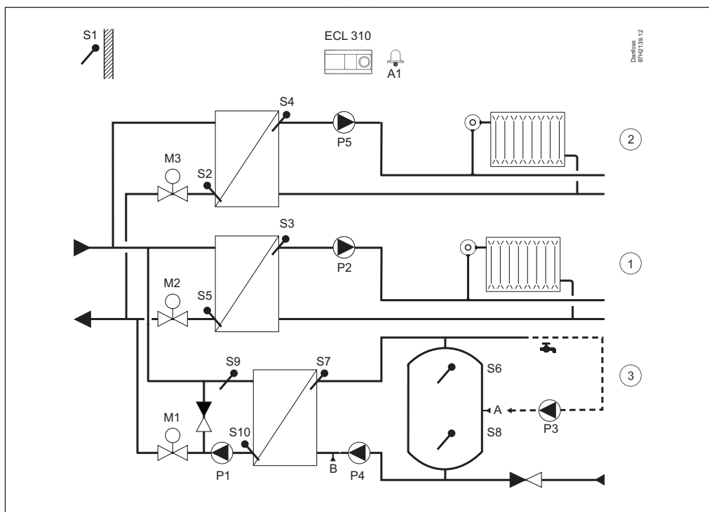
А390.13, приклад А: Два незалежно приєднаних контури опалення та один контур завантаження ГВП. Завжди пріоритет завантаження ГВП.
