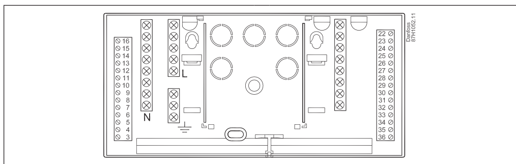
Клемна панель ECL Comfort 210
