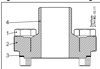
Figure 23: ICFW SS 25 welding module, 25 DIN
