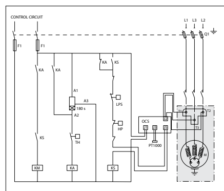
Huzalozási rajz leszivattyúzási ciklus nélkül.
