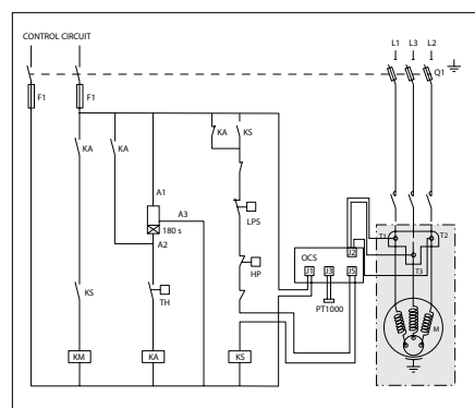
Schaltplan ohne Pump-Down-Zyklus
