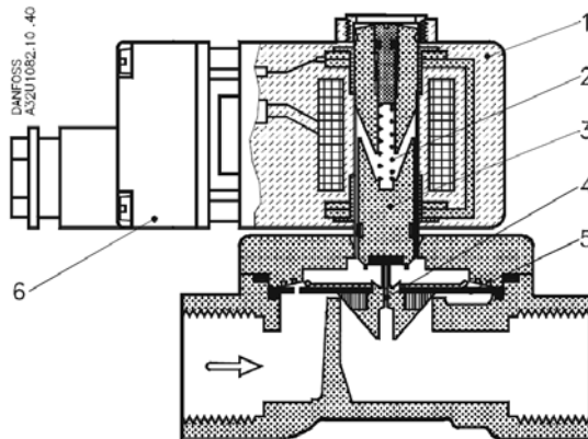
Нормально закрытый пропорциональный электромагнитный клапан.
